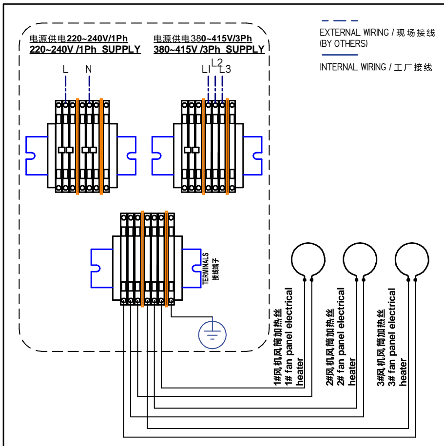
3 风扇/3FANS
