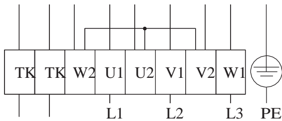
Y: 连接 Y: CONNECTION
