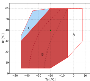
R404A- H33
