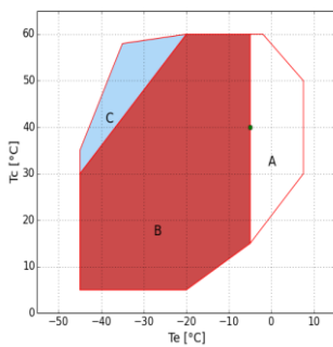
R404A- H33
